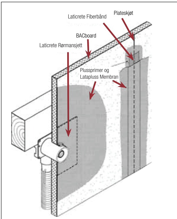
Fig. 2 Prinsipp for tetting rundt rørgjennomføringer og ved skjøter
