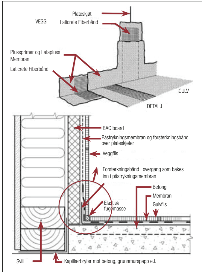
Fig. 3 Eksempel på overgang mellom fliskeidd golv og vegg med membran under flisene på golv.
