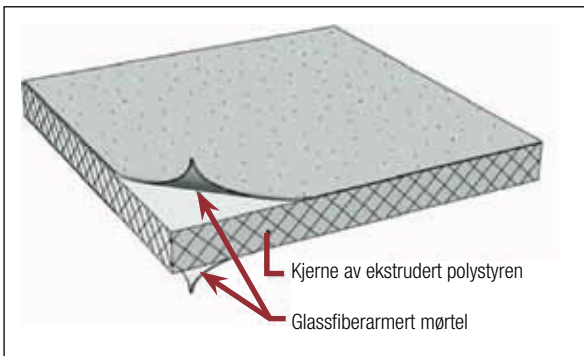
Fig. 1 Oppbygningen av BACboard. Platene er symmetriske med armert mørtel på begge sider.
